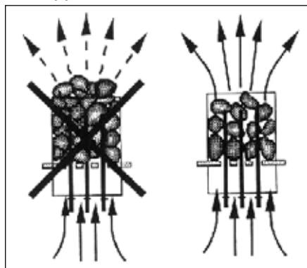
Рис. 1. Укладка камней
